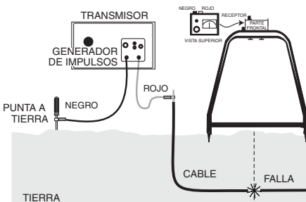
Figura 4. Receptor de Anulación – Primera Vez
