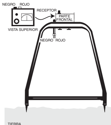
Figura 2. Instalación del Receptor
